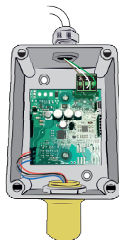
Sonda con sensore nuovo rimontato
