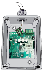
Sonda con sensore smontato
