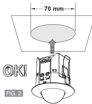
Instalação encastrada em tecto falso
