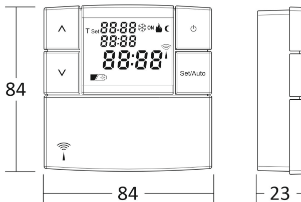
Dimensioni (mm)
